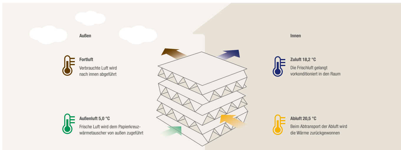
Die Struktur des Lossnay Papierkreuzwärmetauschers
