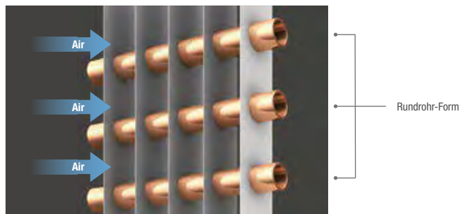
Rundrohr-Wärmetauscher
