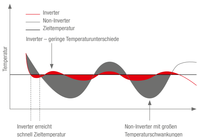
Wirkungsprinzip Inverter
