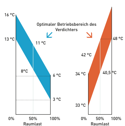
Verdampfungstemperatur Verflüssigungstemperatur
