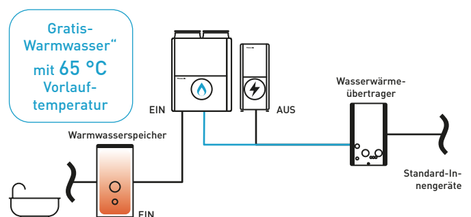
Vorrang für die Brauchwarmwasserbereitung
