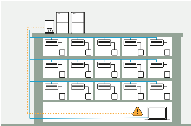
Abb. 1: Kältemittel-Sammelstation von Panasonic
