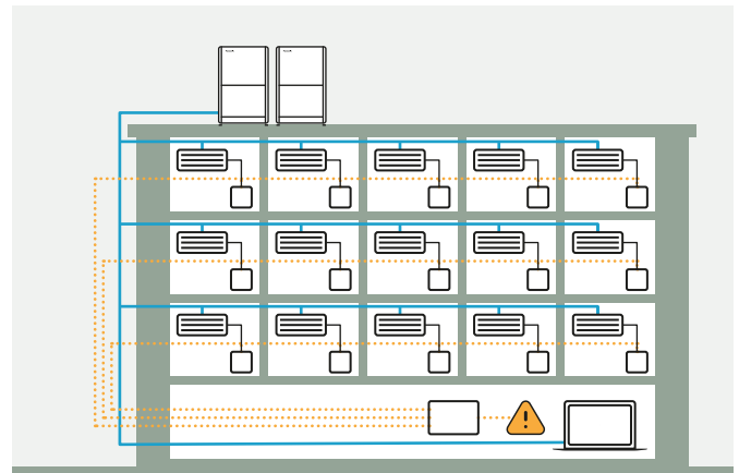
Abb. 2: Herkömmliches, eigenständiges Leakage-Erkennungssystem
