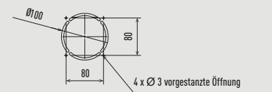
Detailansicht X
