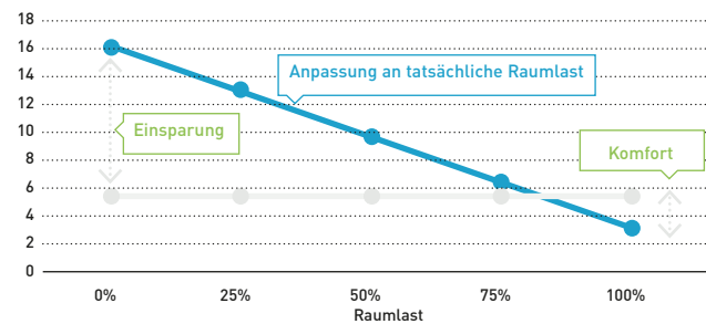
Variable Verdampfungstemperatur
