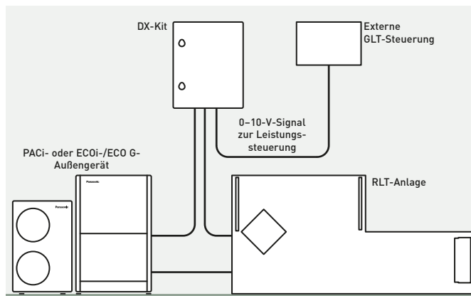
Leistungssteuerung des Außengeräts durch externes 0-10-V-Steuersignal
