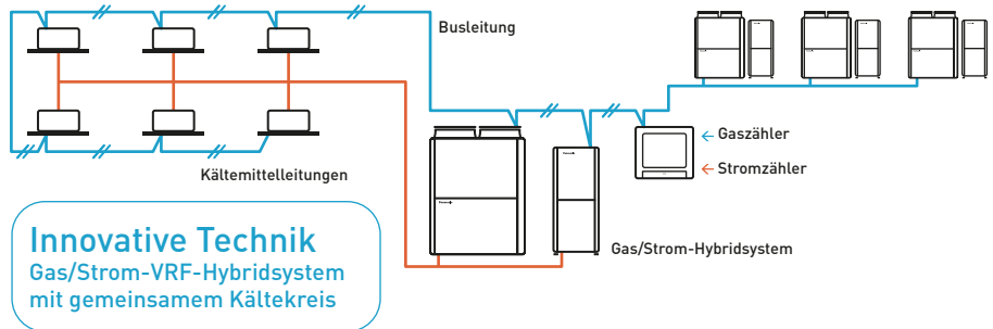
Systembeispiel für Gas/Strom-Hybridsystem
