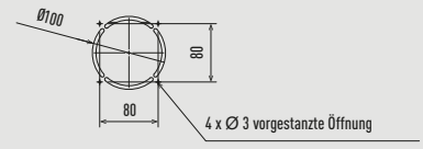
Detailansicht X
