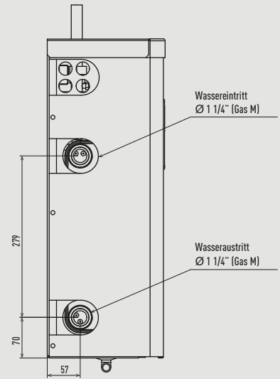
Seitenansicht links
