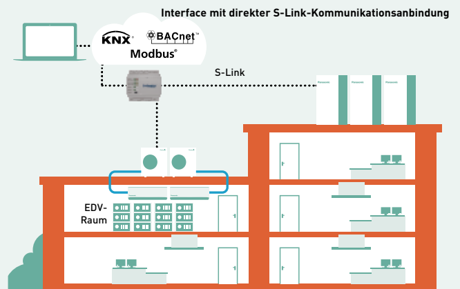
Direkter Anschluss der GLT-Interfaces an S-Link zur Steuerung von bis zu 128 Innengeräten
