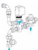
3-Wegeventil für Hauptregister
